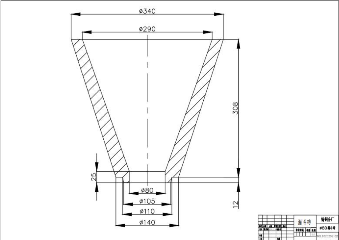
漏斗砖
